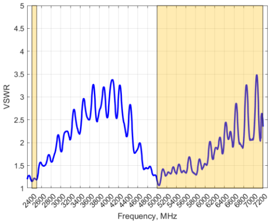
VSWR: WI-FI
